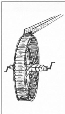
Vasshjul av overfallstype.
