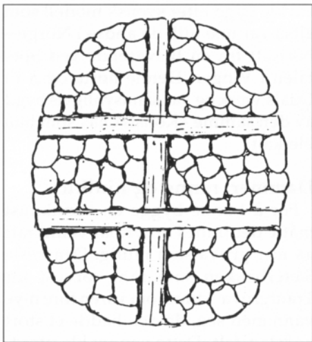
Skisse av hovedfundament for stangfeltet.
